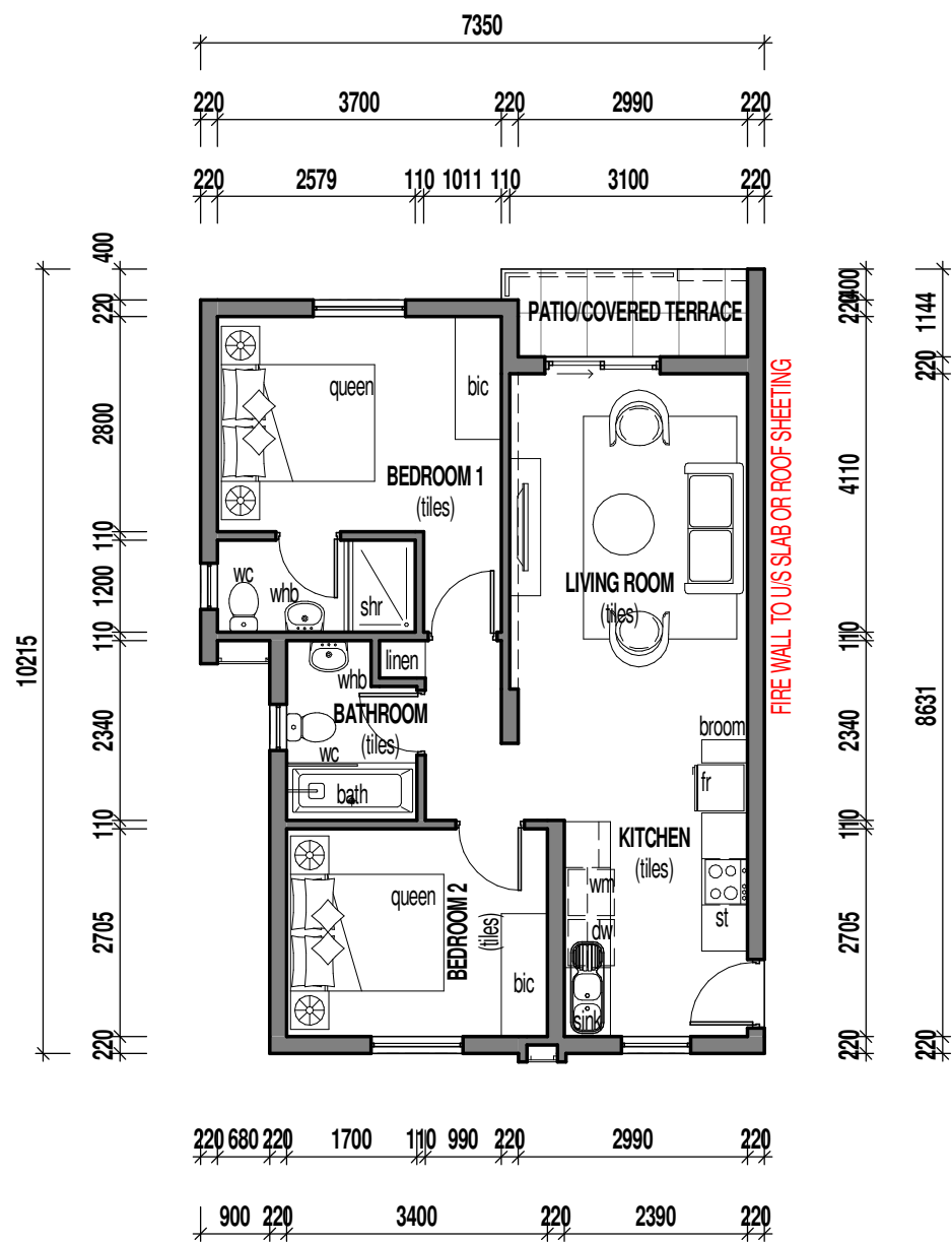
1 UNIT TYPE A 1 : 100
