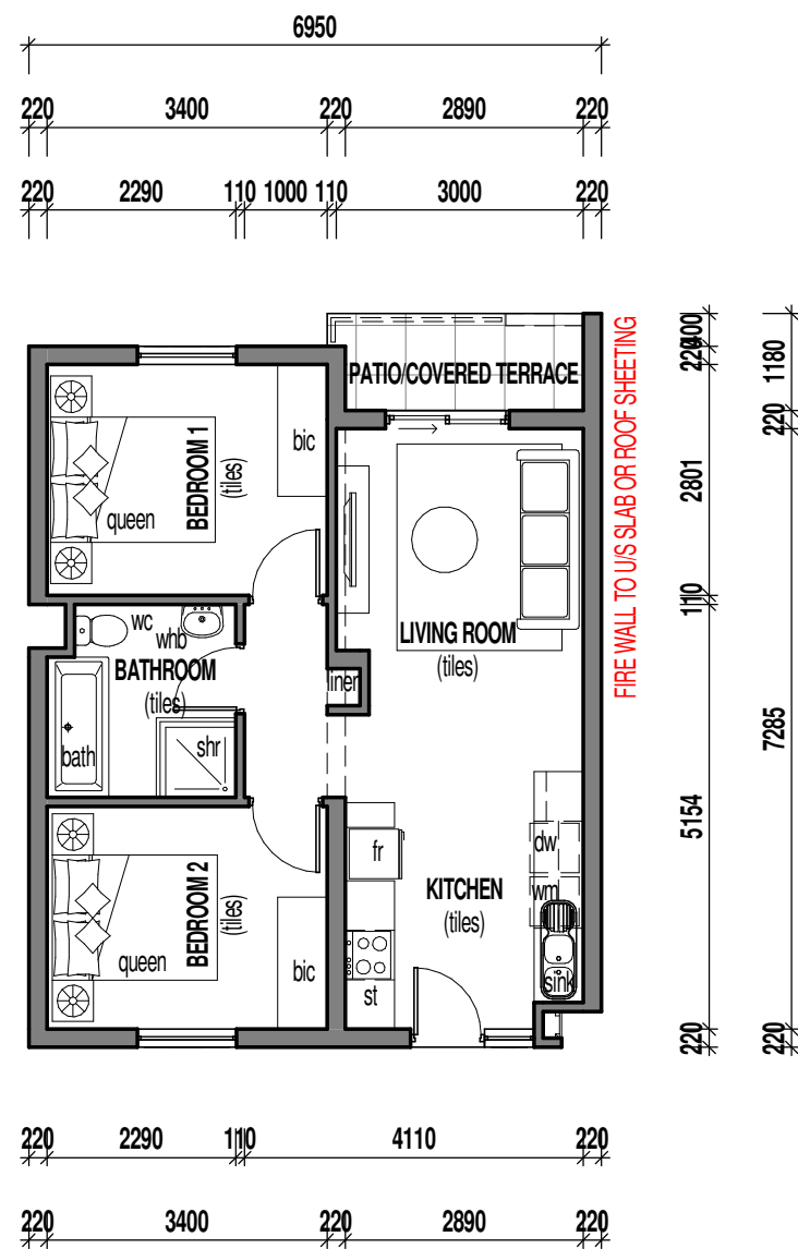
3 UNIT TYPE B1 1 : 100
