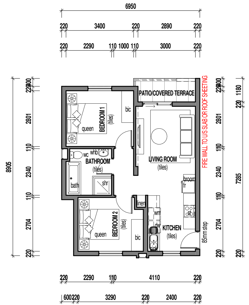
2 UNIT TYPE B 1 : 100
